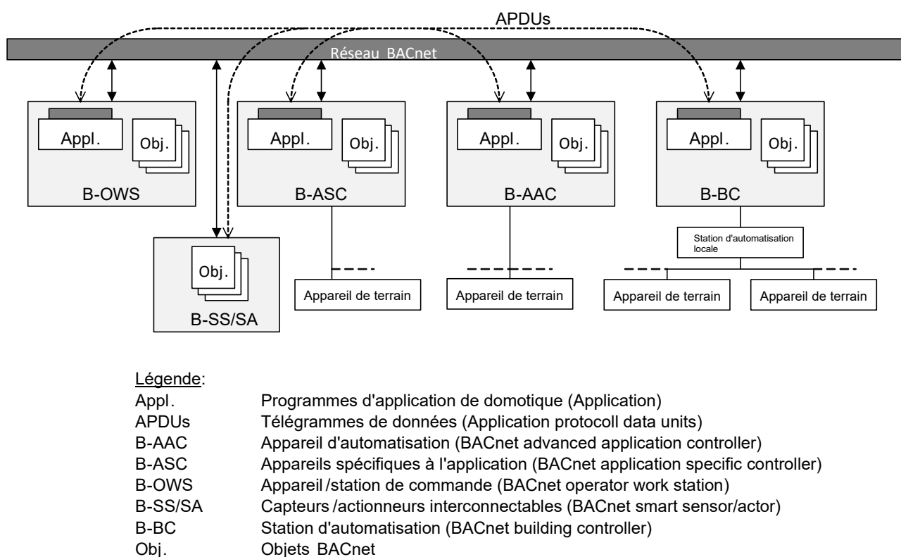
Figure 3: Aperçu de la structuration des systèmes BACnet (selon [4])
