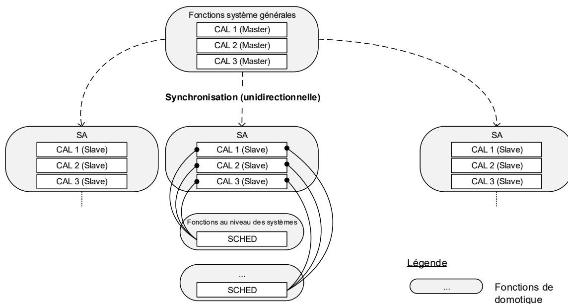
Figure 5: Concept de synchronisation des entrées de calendrier et référence des plans de commutation temporisée à des objets calendrier
