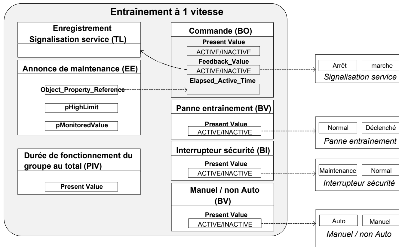
Figure 9: Relation fonctionnelle des fonctions de domotique de l'entraînement à un niveau
